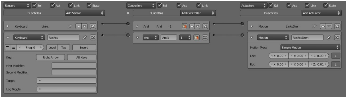
Abb. 3–7 Logic Bricks für die komplette Drehung
