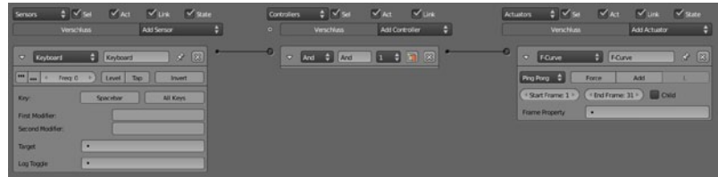
Abb. 3–8 Logic Bricks für den Verschluss
