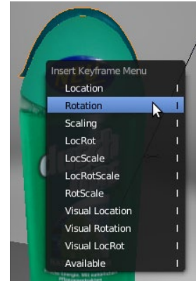
1. Keyframe
