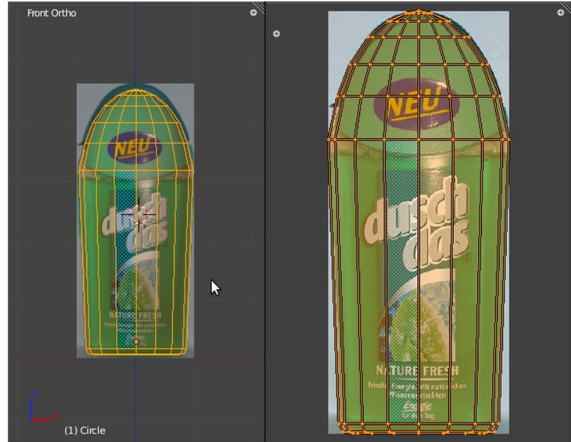
Abb. 3-15 Die Projektion
